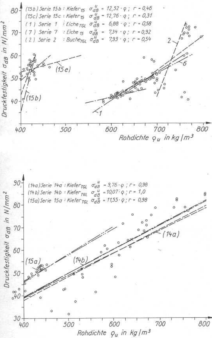
Bild 4. Korrelation zwischen Druckfestigkeit und Rohdichte (eigene Versuche)
