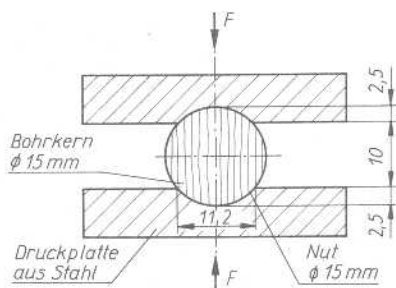
Bild 1. Prinzip der Prüfung von Bohrkernen aus Holz
