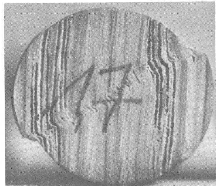
Bild 2. Bruchbilder. a - typischer Bruch der Quader, 20 mm x 20 mm x 30 mm, nach TGL 25 106 (Holzart: Buche); b - typischer Bruch der Bohrkerns parallel zur Faser, Durchmesser 15 mm (Holzart: Eiche)
